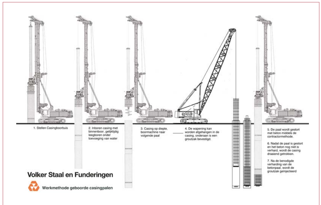
Figuur 2 Beschrijving uitvoering geboorde casingpalen.
