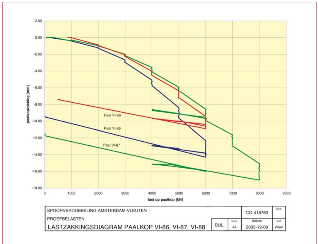
Figuur 4 Resultaat proefbelastingen.
