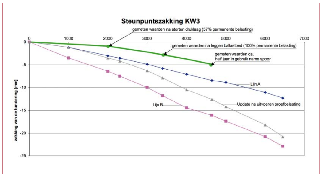
Figuur 5 Aangenomen en geregistreeerde last-zakkingsgedrag steunpunten.
