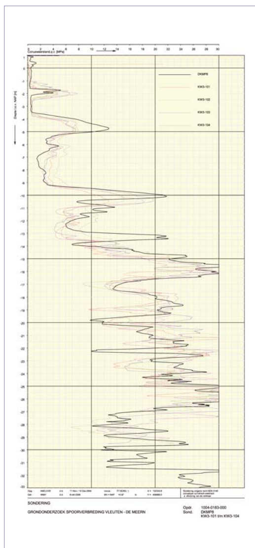
Figuur 3 Resultaat sonderingen vóór en na paalinstallatie.
