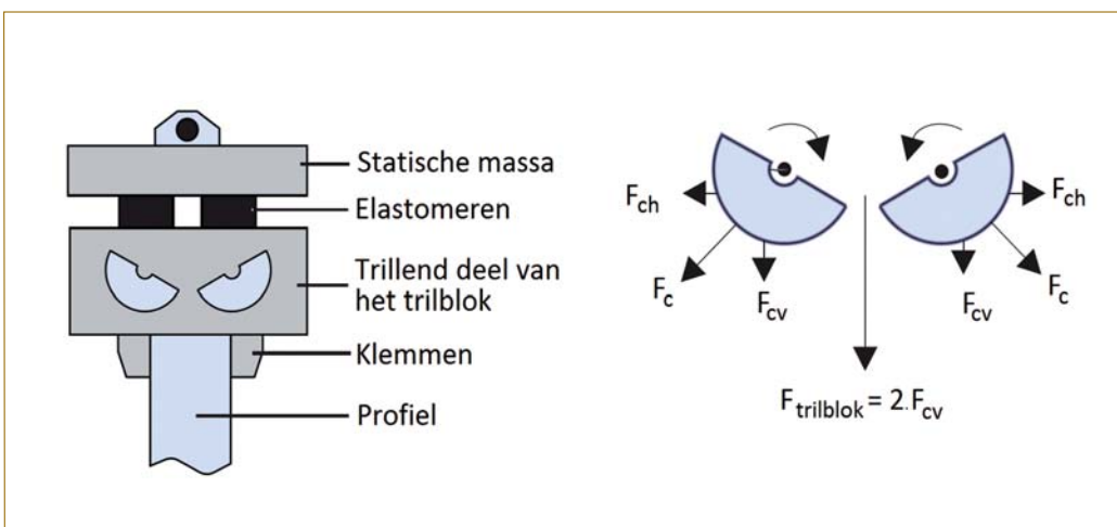
Figuur 2 - Algemeen principe van de triltechniek [10].
