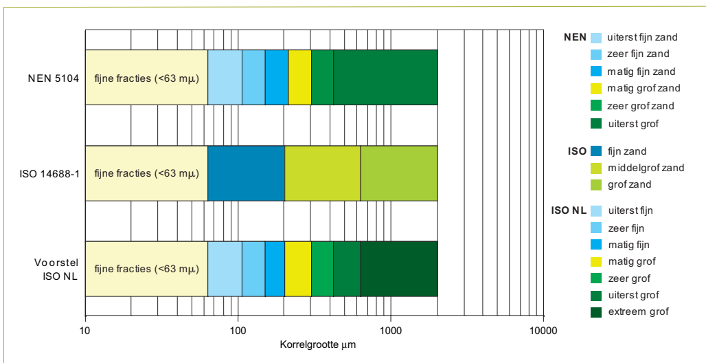
Figuur 2 – Onderverdeling zandfracties volgens NEN 5104, ISO 14688-1 en voorstel Nationale Annex.
