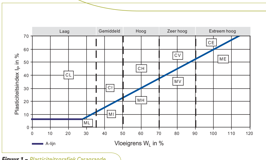
Figuur 1 - Plasticiteitsgrafiek Casagrande.
